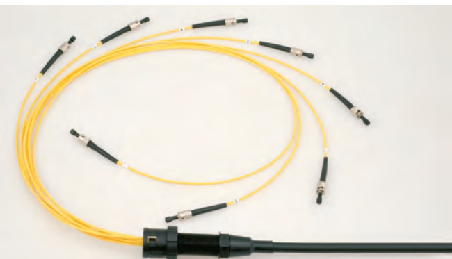
04 Cables minibreakout escalonados para una fácil inserción en cajas de empalmes preparadas. Además, los cables minibreakout están codificados con números
