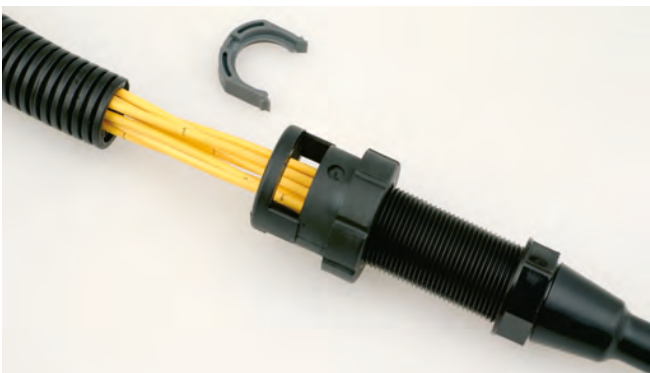
03 Vista detallada del cuerpo divisorio fundido. Está equipado con un prensaestopas PG compatible para la instalación en cajas de empalmes de HELUKABEL®. Además, el sistema se puede reutilizar cuando se reubica.
